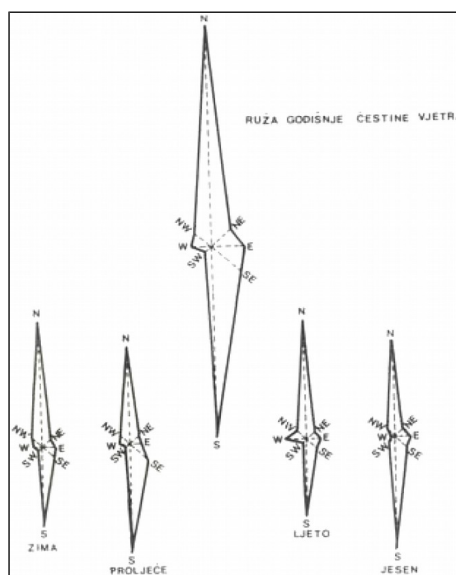
Slika 6. Ruža vjetrova
